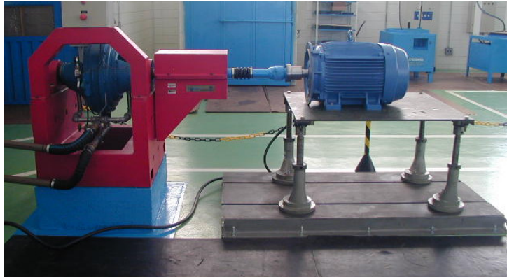
DINAMÔMETRO
